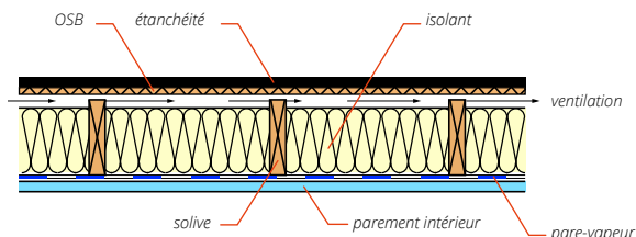
Toitures terrasses « froides » standard avec la difficulté d'assurer une bonne ventilation, augmentant le risque de condensation au niveau des éléments en bois (solives, panneaux bois support de l'étanchéité). ©AQC
